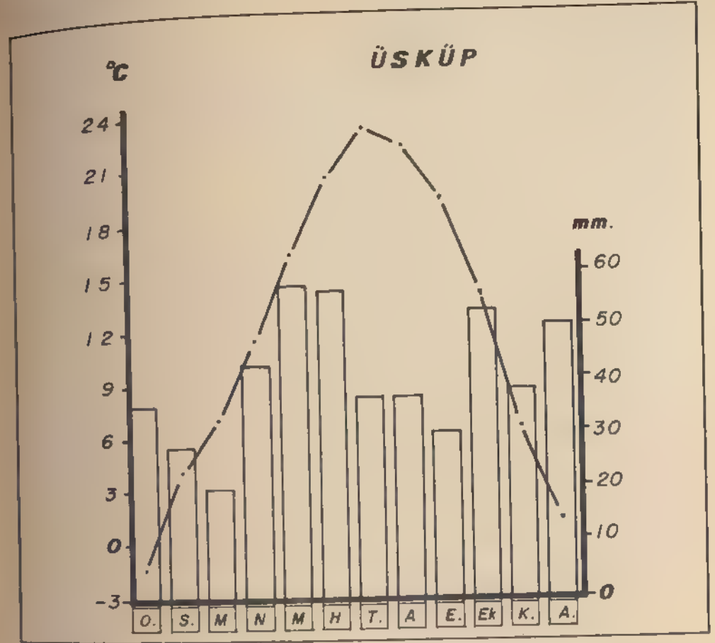
Şekil 13- Üsküp'un iklim diyagramı. Sıcaklık kesik çizgi ile, yağış sütunlarla gösterilmiştir.
